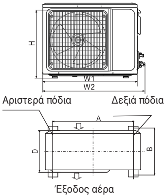
Βίδα εγκατάστασης εξωτερικής μονάδας
